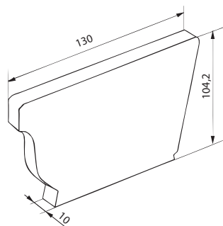
Заглушка левая
