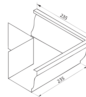
Угол внешний 90°
