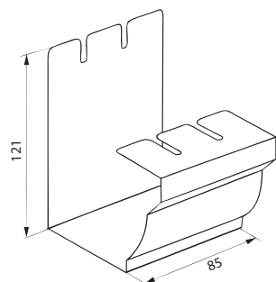
Соединитель желоба
