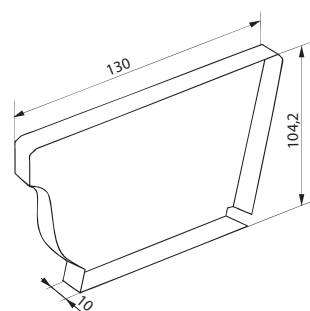
Заглушка правая
