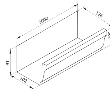
Прямоугольный желоб
