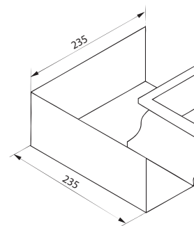
Прямоугольный желоб
