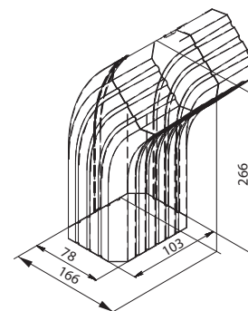
Угол внутренний 90°
